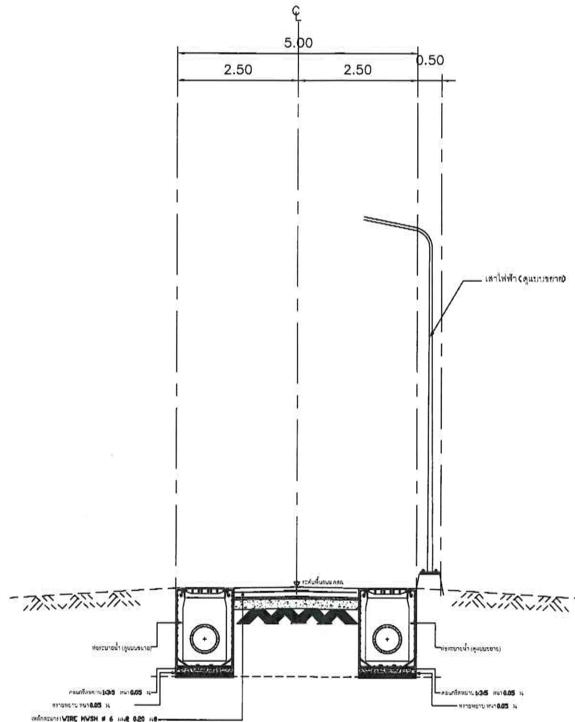
แบบรูปตัด ถนนกว้าง 5.00 ม.
