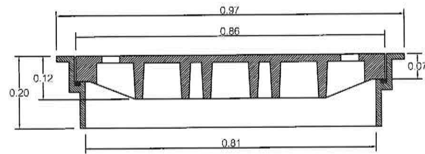
รูปตัดตามขวางฝาบ่อพัก
