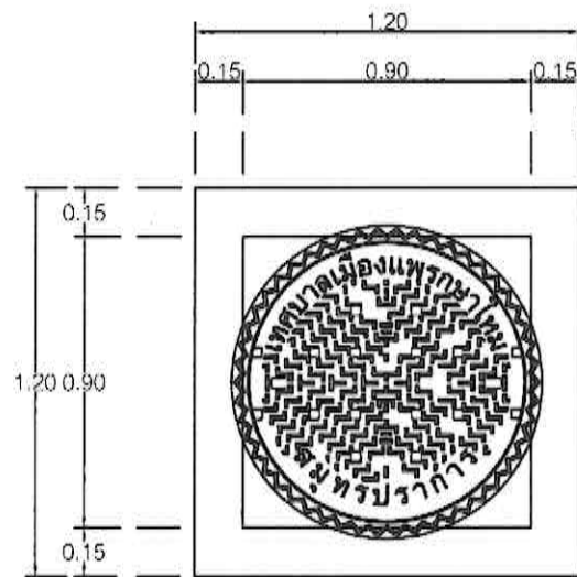
แบบแปลนบ่อพักท่อระบายน้ำ 1 : 25
