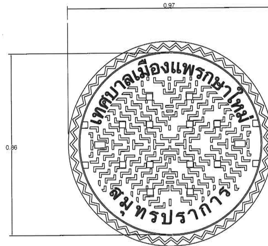
แปลนฝาบ่อพักบน
