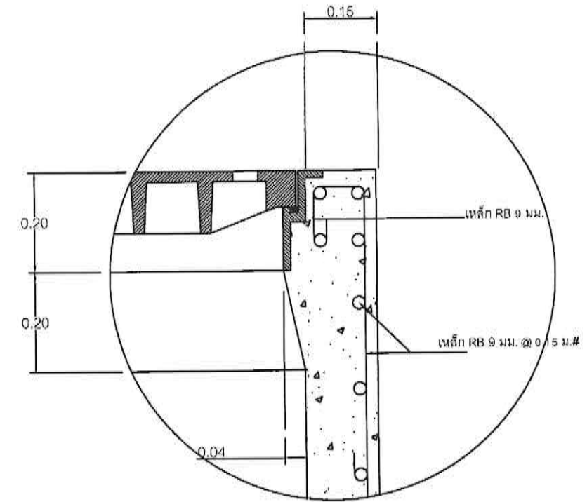
ขยายบ่อรับฝาบ่อพัก
