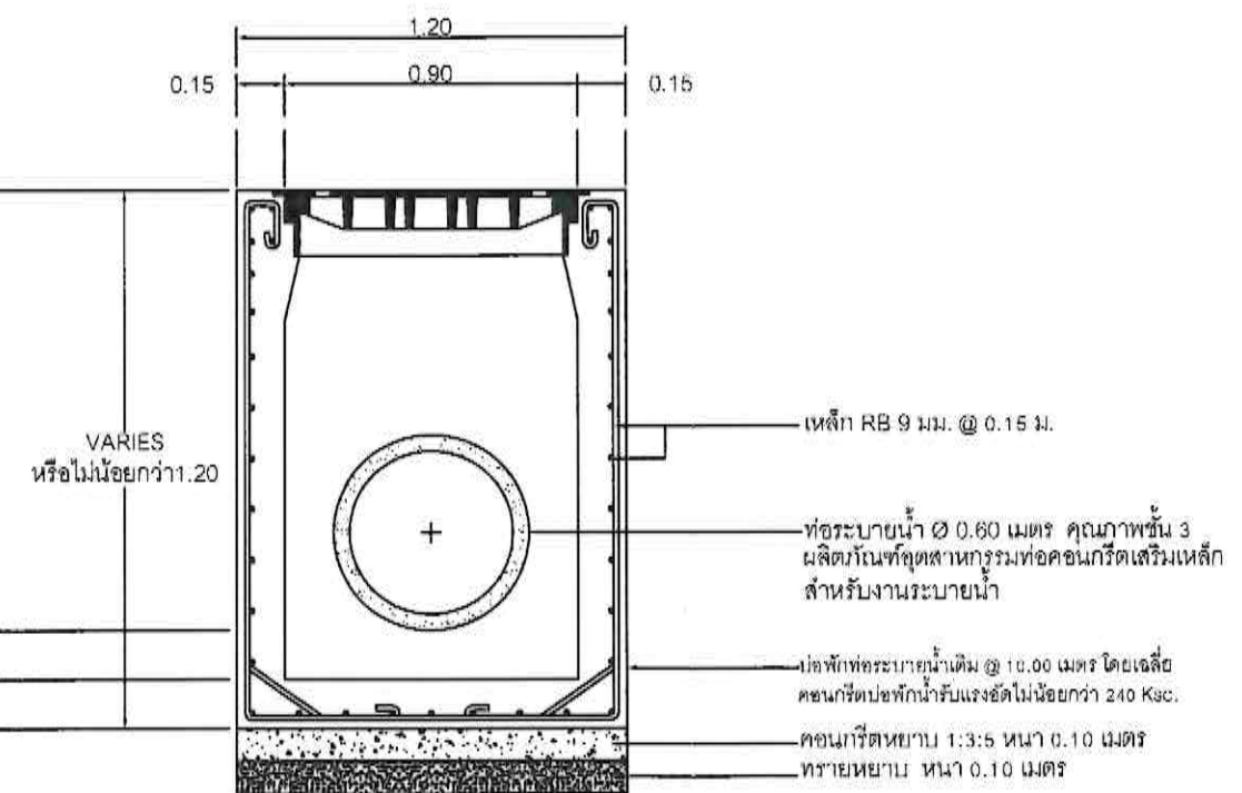
รูปตัดท่อระบายน้ำ 1 : 25
