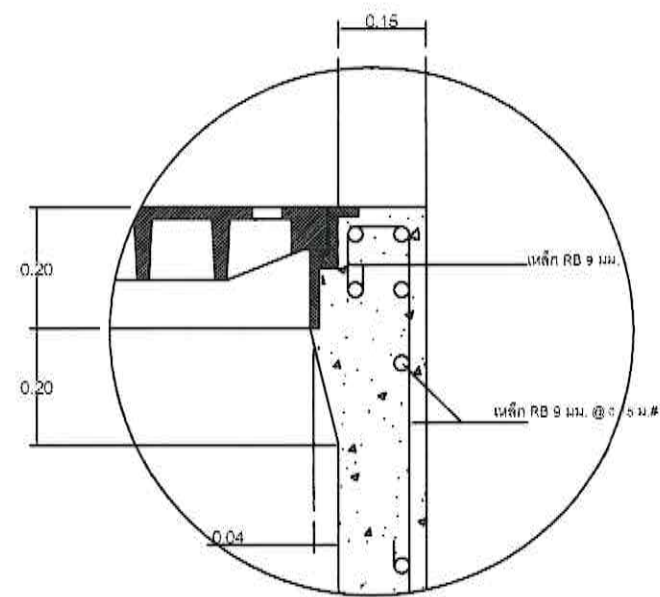
ขยายบารับฝาบ่อพัก 1 : 25
