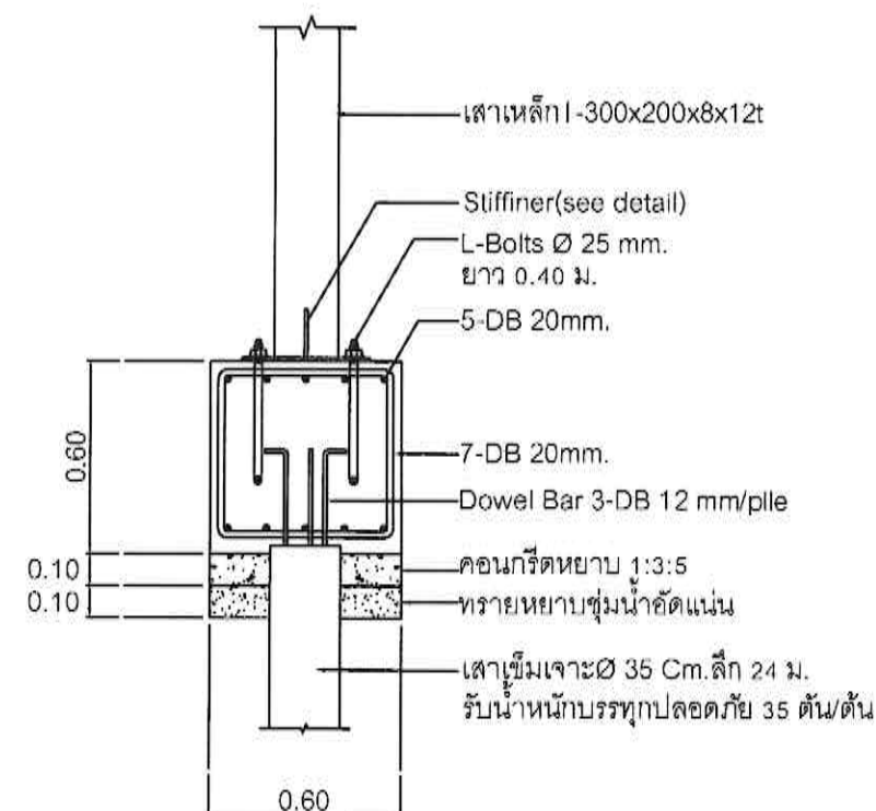
รูปตัดฐานราก B-B 1 : 25
