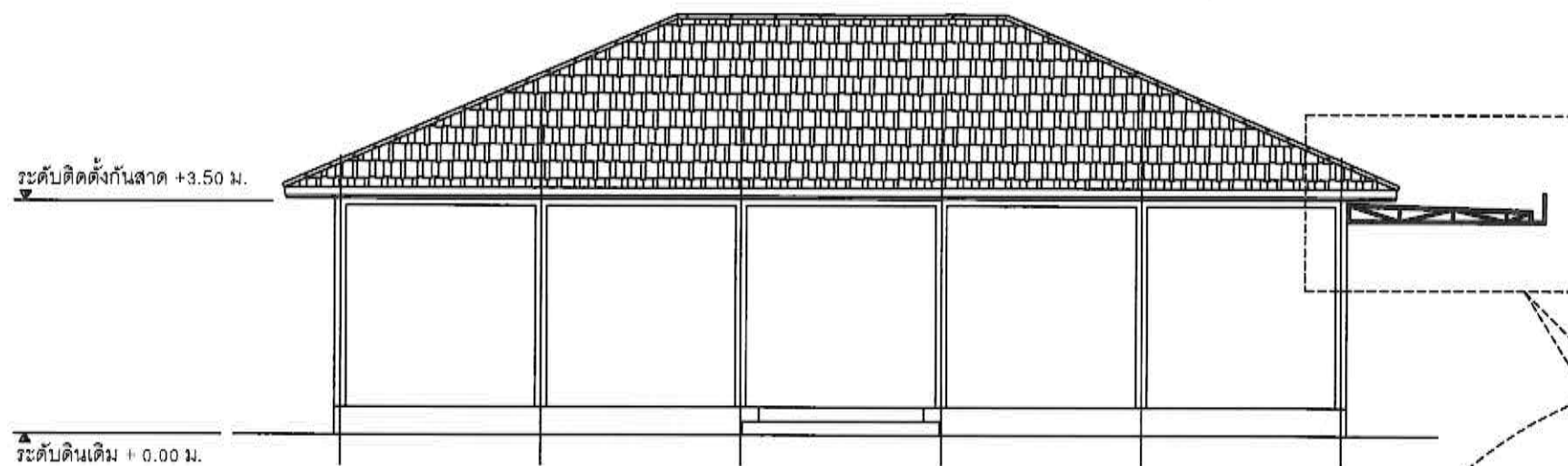
รูปด้าน 1 1:100
