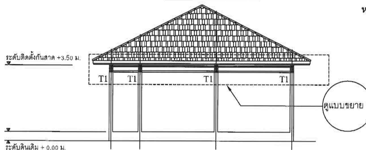
รูปด้าน 2 1:100
