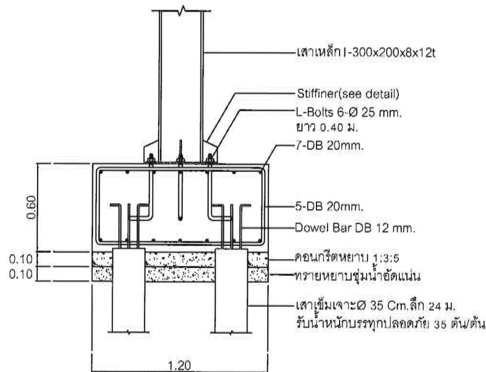
รูปตัดฐานราก A-A 1 : 25
