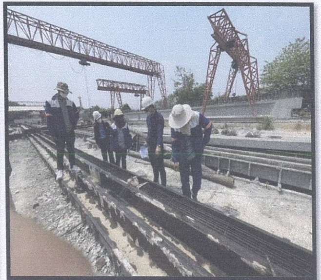
ภาพถ่าย ขั้นตอนการตรวจสอบโรงงานผลิตเสาเข็ม ค.ส.ล.ขนาด 0.26 x 0.26 เมตร
